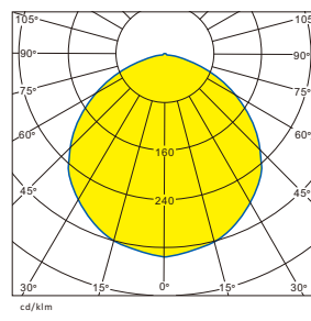
NEMA 7H7V for 30W~155W
